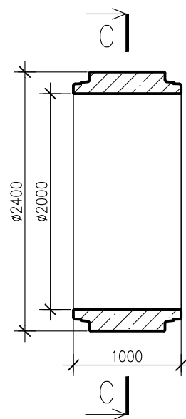
PRZEKRÓJ C-C
